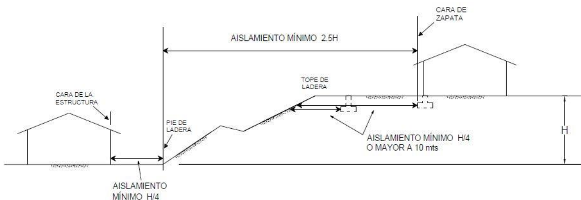
Figura 6.2.12-1 — Distancia mínima para ubicación del proyecto desde el borde del barranco [1]
